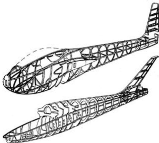
Slika 3: Trup zrakoplova
