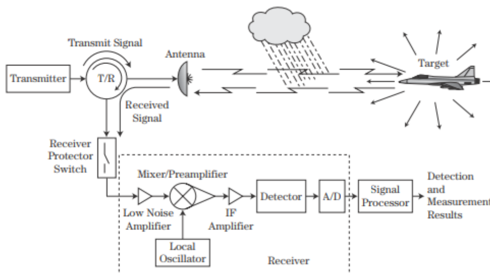
Slika 1 Shema važnih dijelova radara [1]
