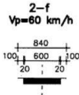
Slika 23. Tipski poprečni presjek ceste
