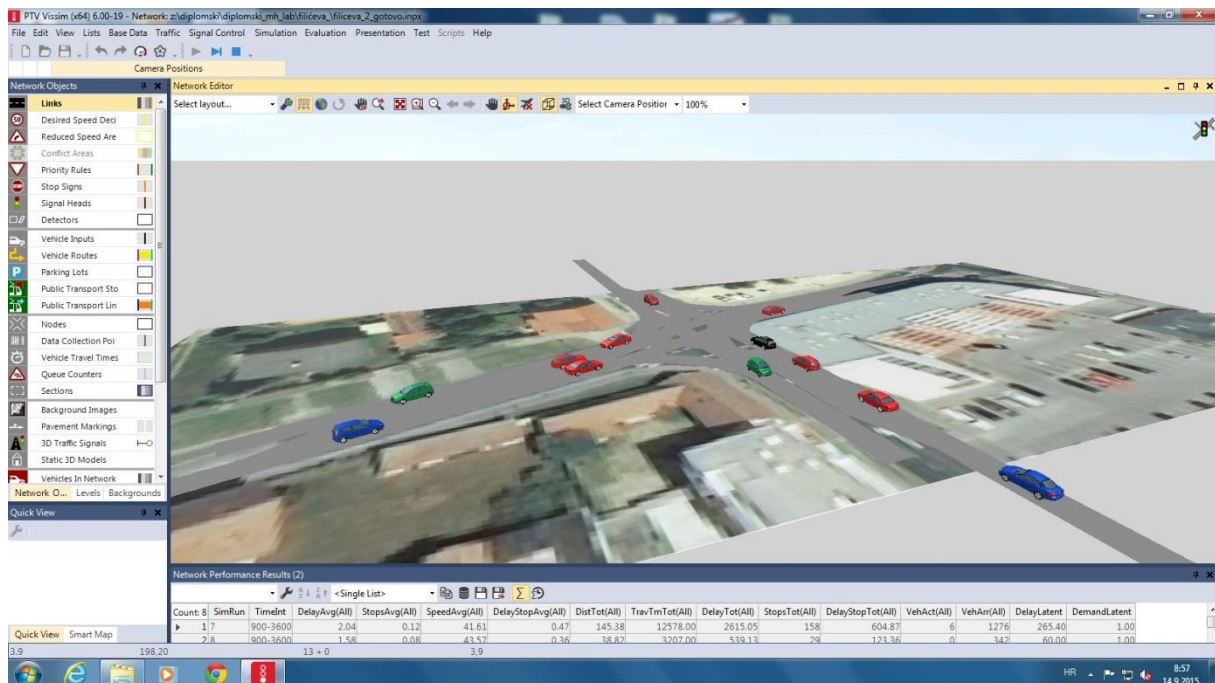
Slika 34. Simulacija postojećih prometnih tokova raskrižja Ulice K. Filića i M. Krleže
