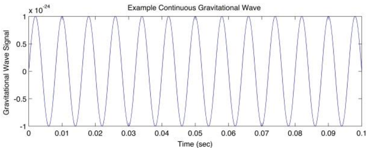
Slika 2.1.2: Kontinuirani val [16]
