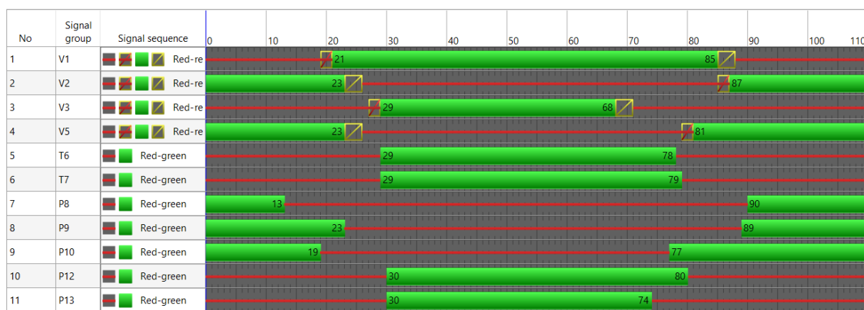
Slika 38. Novi signalni plan raskrižja Ulica kneza Višeslava - Avenija Marina Držića - Šubićeva ulica
