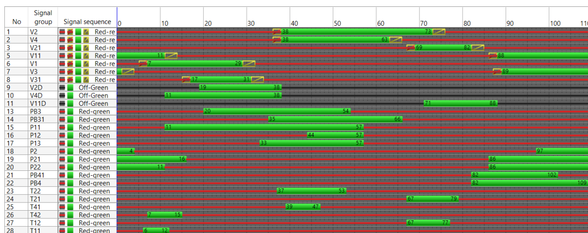
Slika 36. Novi signalni plan raskrižja Ulica kneza Branimira - Avenija Marina Držića
