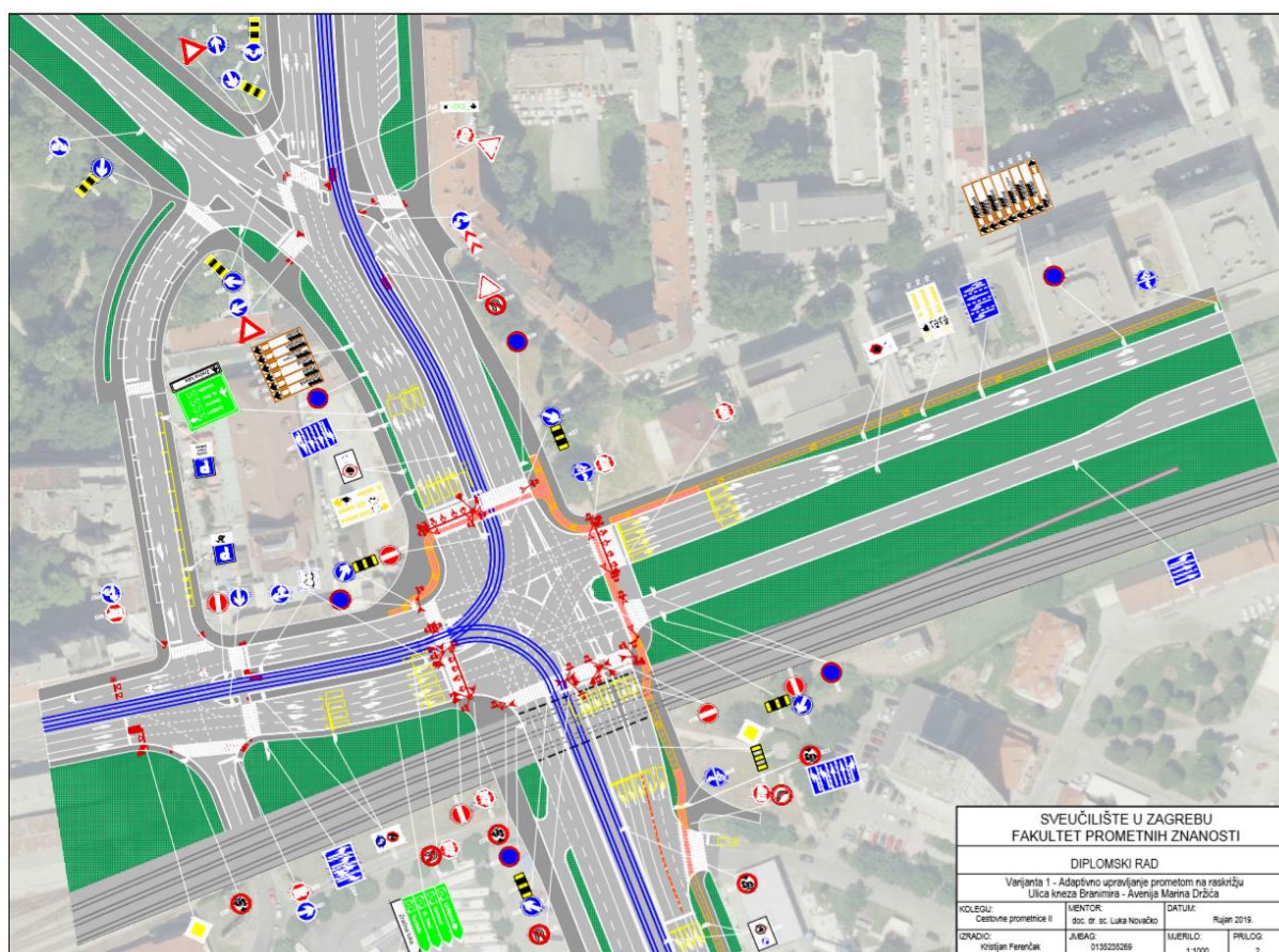
Slika 34. Varijanta 1 - Adaptivno upravljanje prometom na raskrižju Ulica kneza Branimira - Avenija Marina Držića
