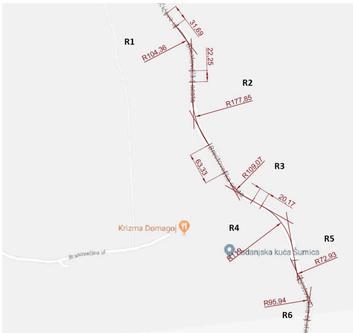
Slika 30. Prikaz duljina pravaca i iznosa radijusa zavoja
