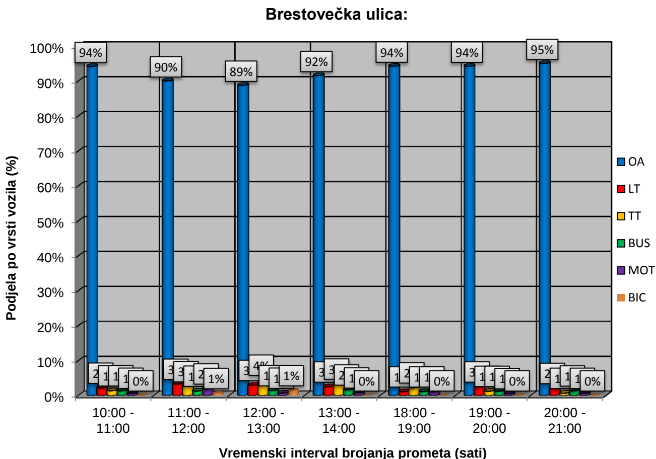
Grafikon 8. Prikaz opterećenja preraspodijeljen po vrsti vozila
