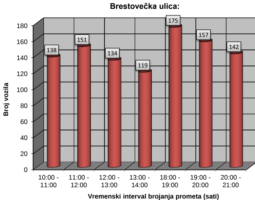
Grafikon 6. Ukupan broj vozila u određenim vremenskim intervalima
