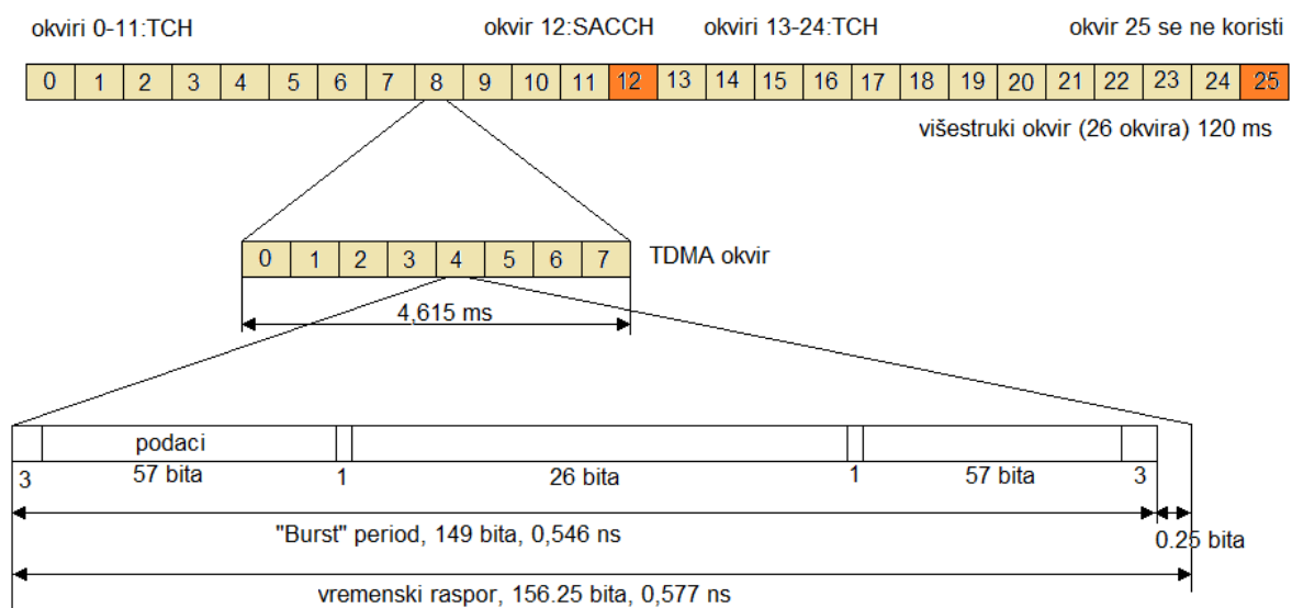
Slika 18. Struktura okvira,
