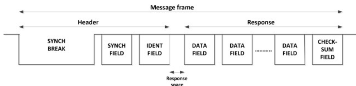
Slika 3.2. LIN protokol[12]
