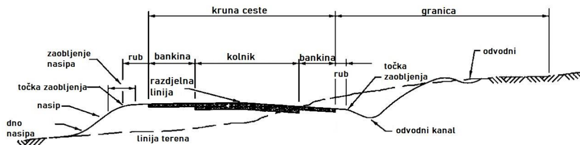
Slika 4. Poprečni presjek ceste
