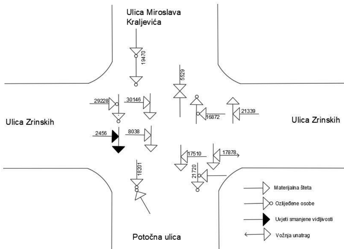
Slika 38. Kolizijski dijagram
