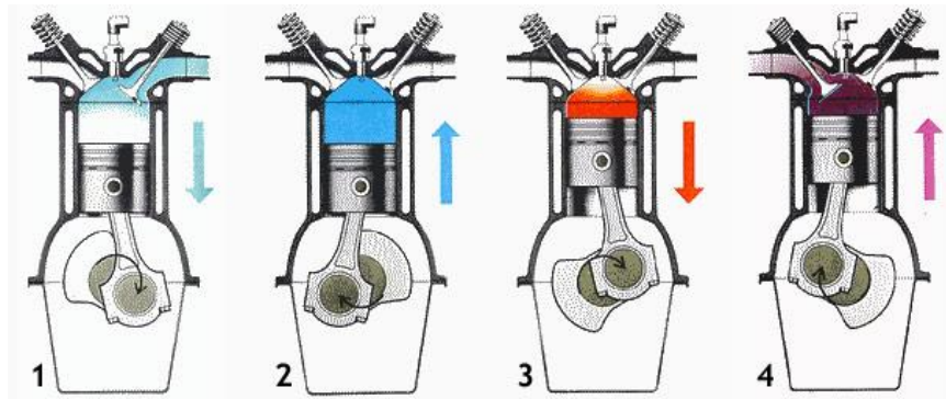
Slika 2. princip rada četverotaktnog motora [9]
