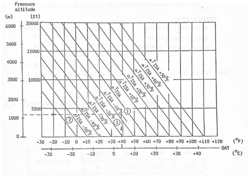
Slika 7 Promjena temperature o visini [1]
