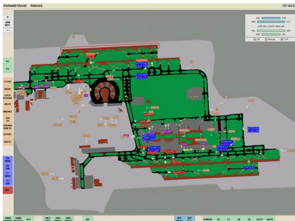
Slika 8. A-SMGCS sustav na monitorima kontrolora [13]
