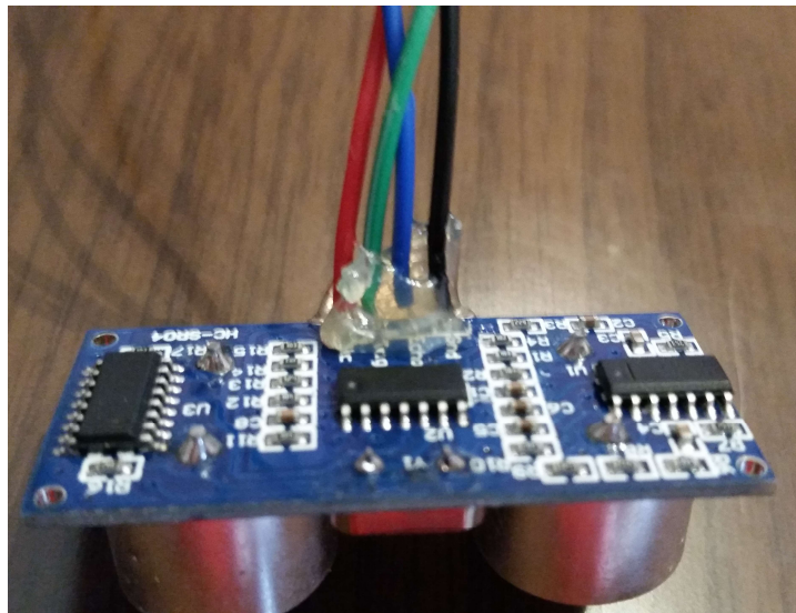
Slika 19 Zalemljeni vodiči ojačani vrućim ljevilom
