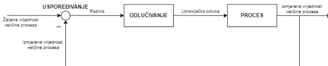
Slika 1: Regulacijska petlja [4]
