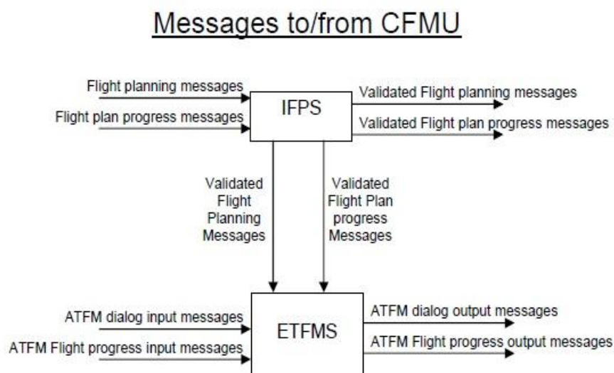
Slika 19. Tok poruka, [46]
