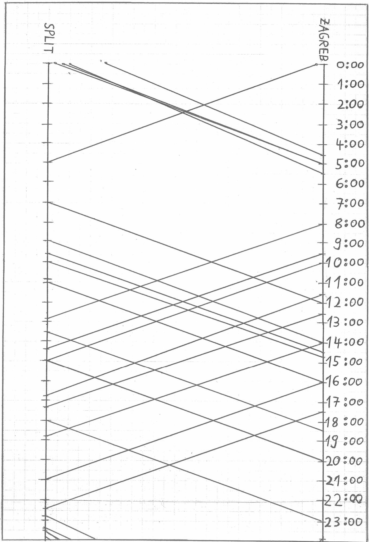
Prilog 4. Grafički vozni red linije 2
