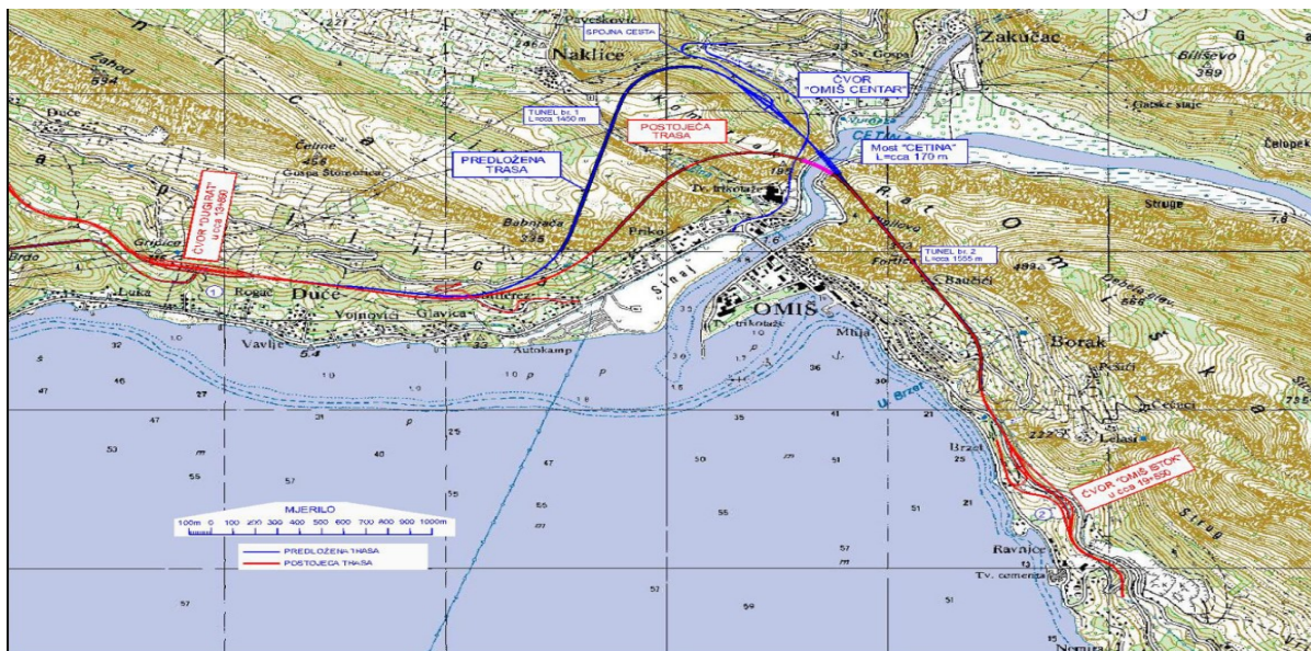
Slika 4. Obilaznica Omiš – Prijedlog korekcije trase ceste
