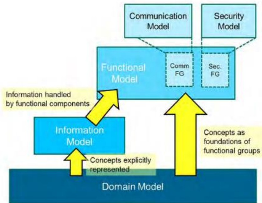
Slika 9. IoT ARM, [31]
