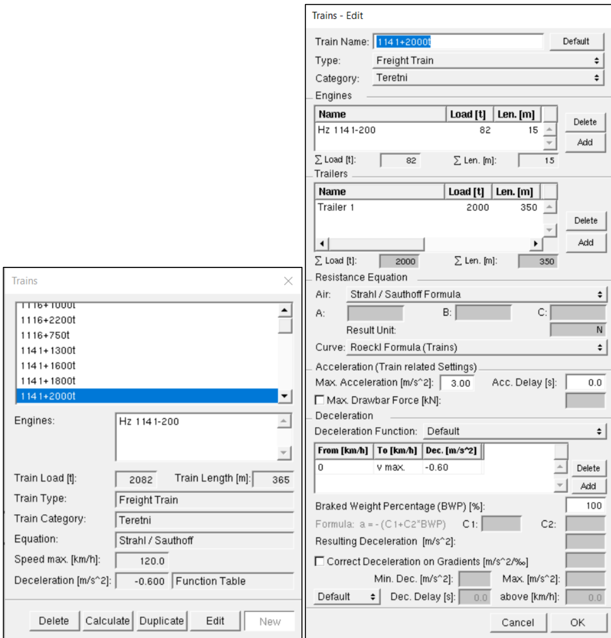
Slika 15. Prikaz izbornika Trains i Trains-Edit u OpenTracku
