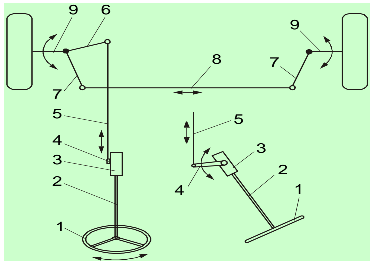
Slika 4.6. Upravljački mehanizam
