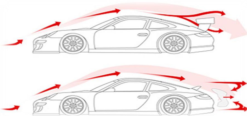
Slika 4.12. Djelovanje usmjerivača zraka
