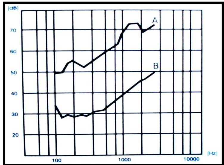
Grafikon 6. Smanjenje buke akustičnom izolacijom
