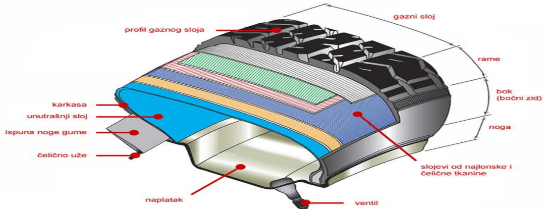
Slika 4.4. Konstrukcija pneumatika
