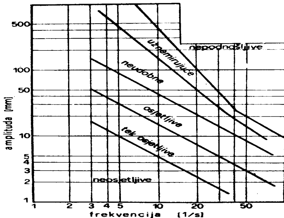
Grafikon 7. Prikaz utjecaja vibracije na čovjeka
