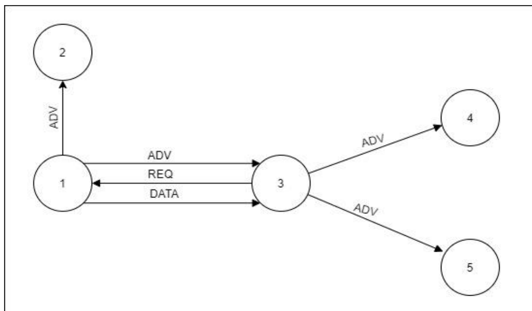
Slika 26. SPIN protokol
