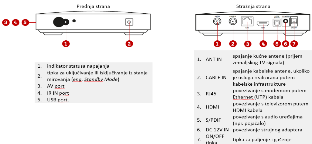
Slika 12. STB Kaon4020
