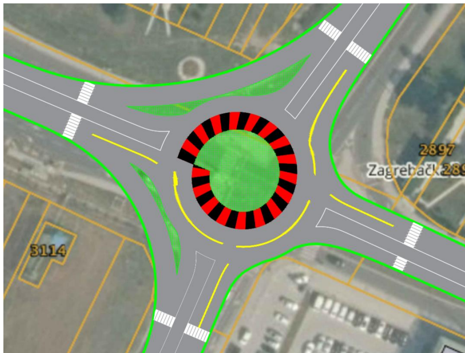
Slika 31. Idejno rješenje prijedloga poboljšanja četverokrakog semaforiziranog raskrižja u koljenasto kružno raskrižje
