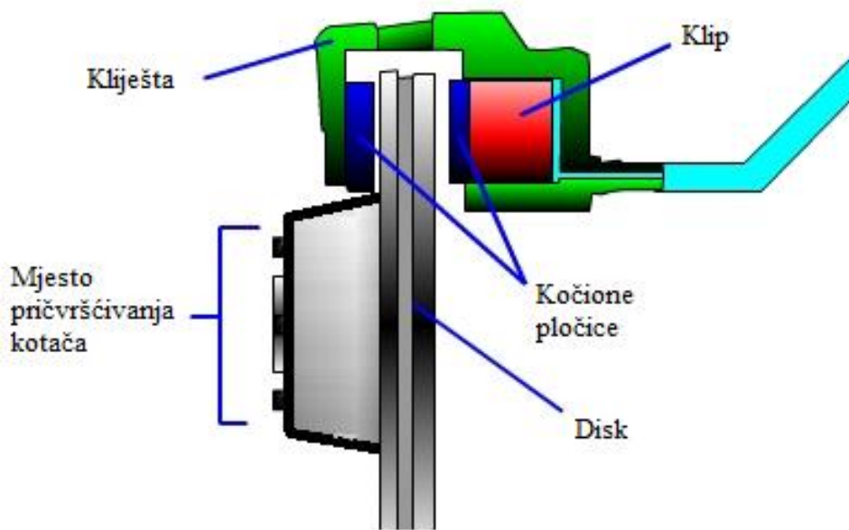
Slika 9. Disk kočnica
