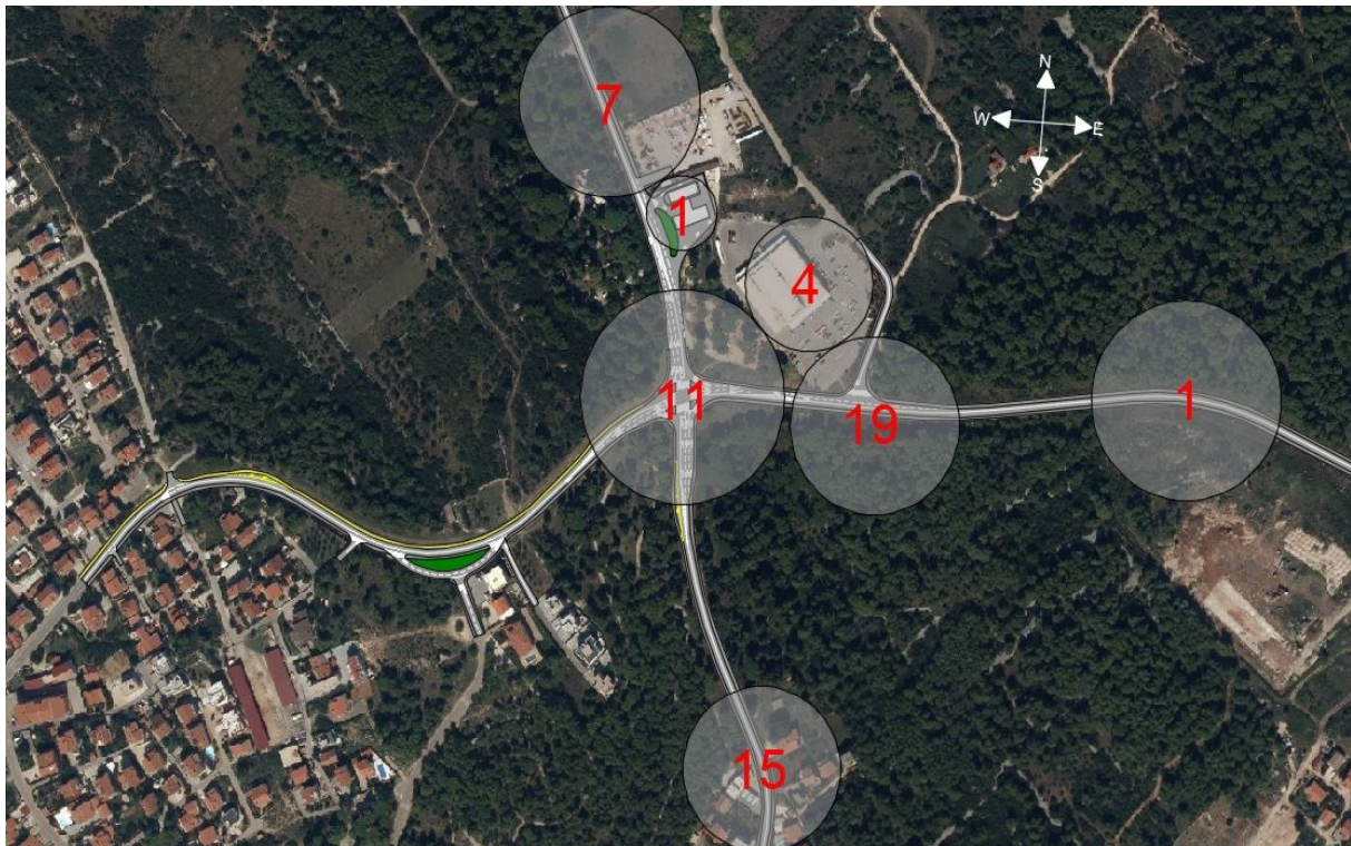
Slika 3.13. Grupiranje i broj prometnih nesreća unutar uže zone obuhvata
