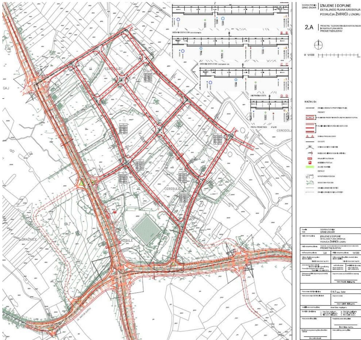
Slika 3.5. Detaljni plan uređenja područja „Žmirići“ u Zadru
