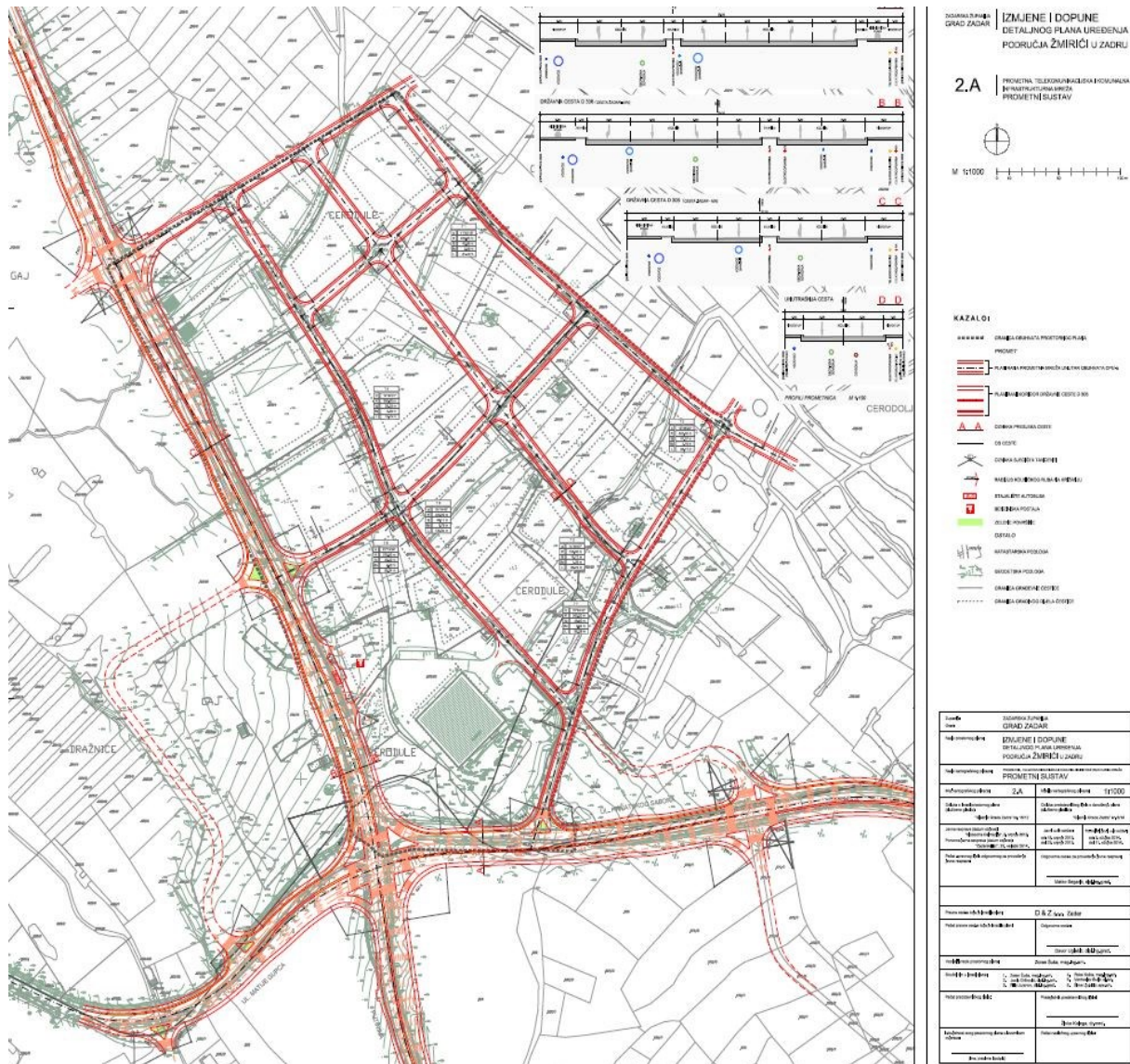
Slika 3.5. Detaljni plan uređenja područja „Žmirići“ u Zadru
