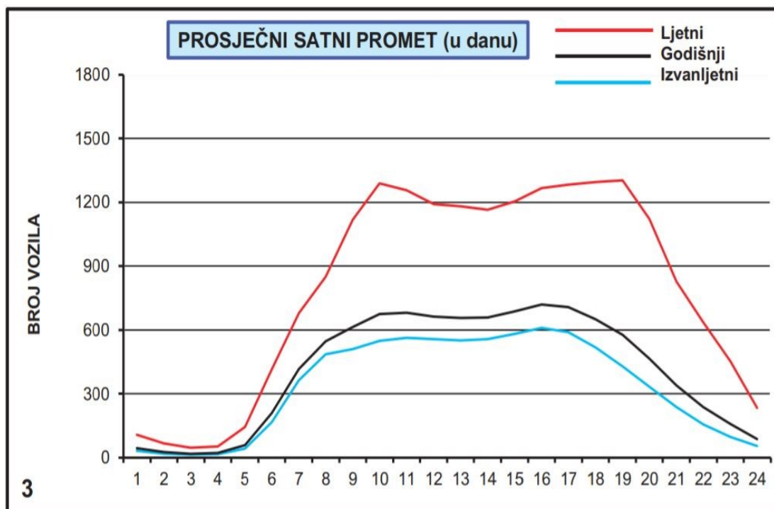
Grafikon 3.4. Prosječni satni promet u danu
