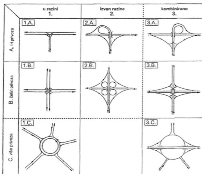
Slika 2.1. Podjela raskrižja
