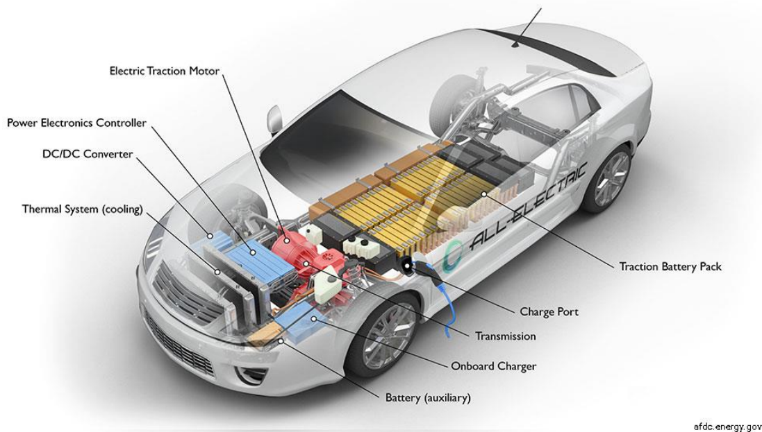
Slika 3. Konfiguracija baterijskog električnog vozila
