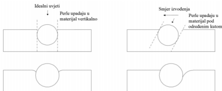
Slika 28. Različiti kut utisnuća kuglica u oznaku
