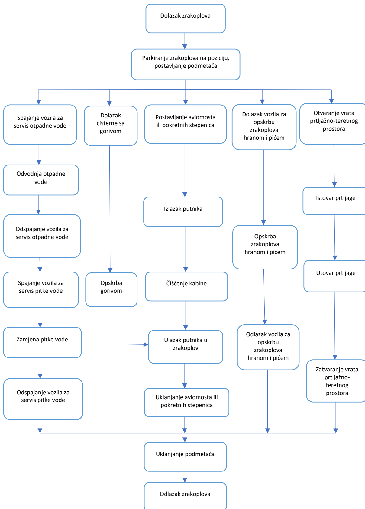
Dijagram 1: Redoslijed aktivnosti u procesu prijema i otpreme zrakoplova redovitog zračnog prijevoznika
