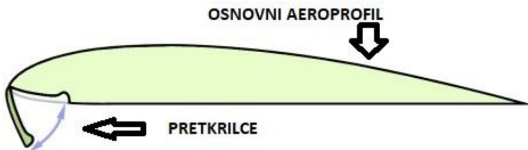
Slika 14. Krugerovo pretkrilce
