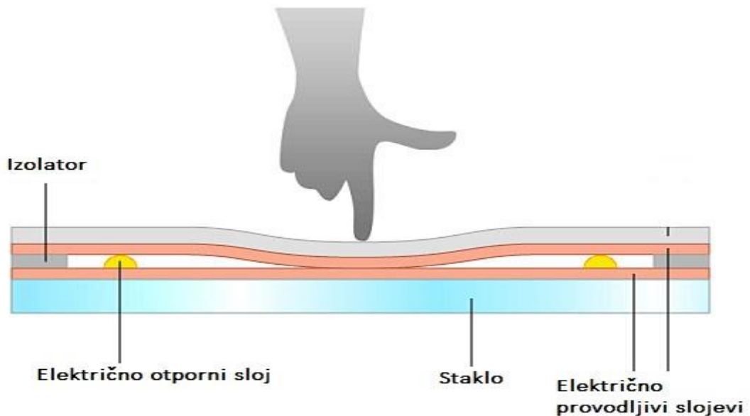
Slika 10. Princip rada zaslona osjetljiv na dodir temeljen na električnom otporu.
