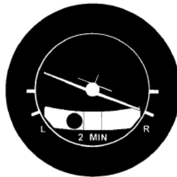
Slika 9. Avion u desnom nekoordiniranom zaokretu Izvor: [2]
