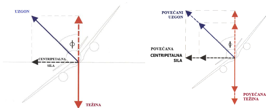
Slika 3. Povećanje sila u zaokretu
