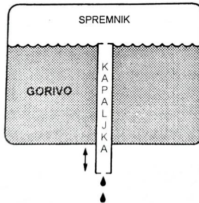
Slika 2. Mehanički mjerač s kapaljkom
