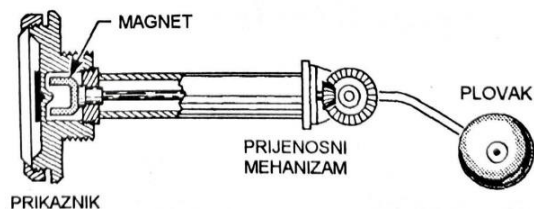
Slika 7. Mjerač s plovkom i magnetnim prijenosom
