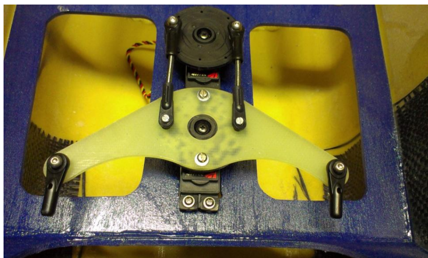
Slika 40. Prikaz ugradnje servo-uređaja za kormilo smjera
