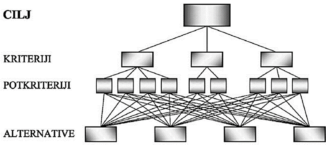
Slika 18. Hijerarhijska struktura AHP metode [54]
