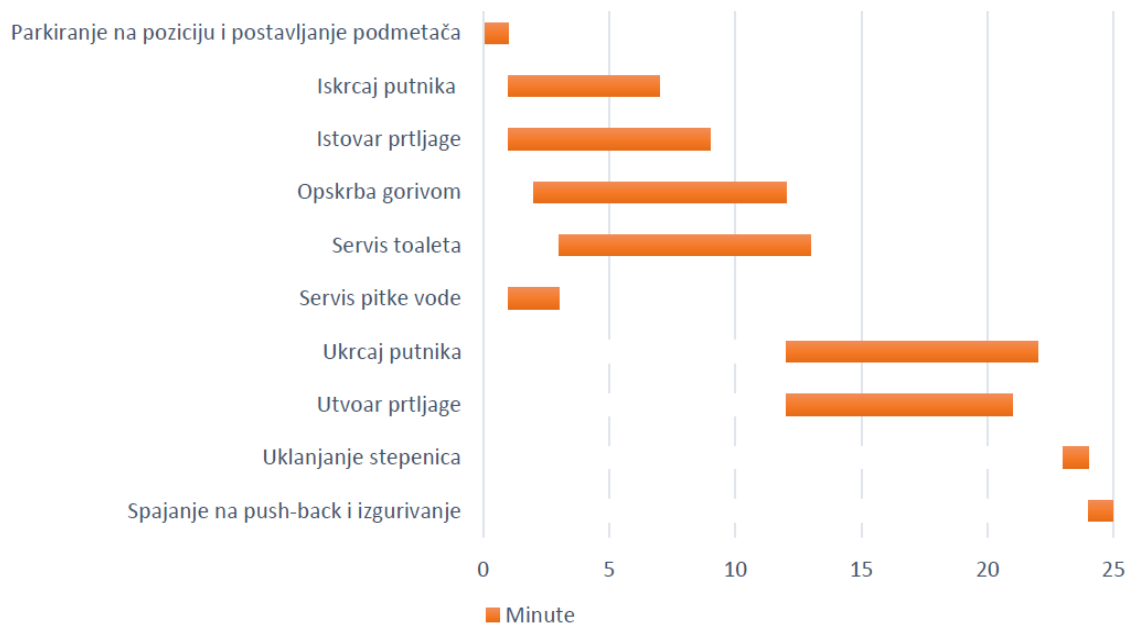
Slika 26. Prikaz aktivnosti minimalnog vremena prihvaata i otpreme B737-800 prijevoznika Ryanair, [15]
