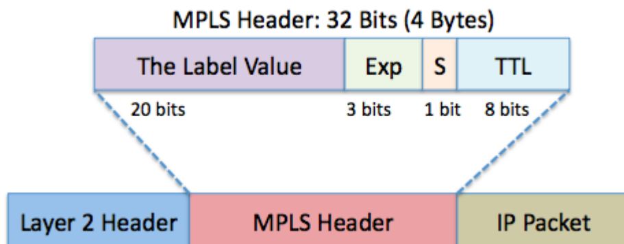
Slika 2 Prikaz MPLS zaglavlja, [8]
