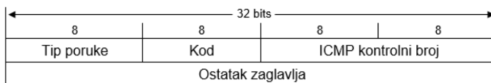
Slika 9 Prikaz formata ICMP zaglavlja
