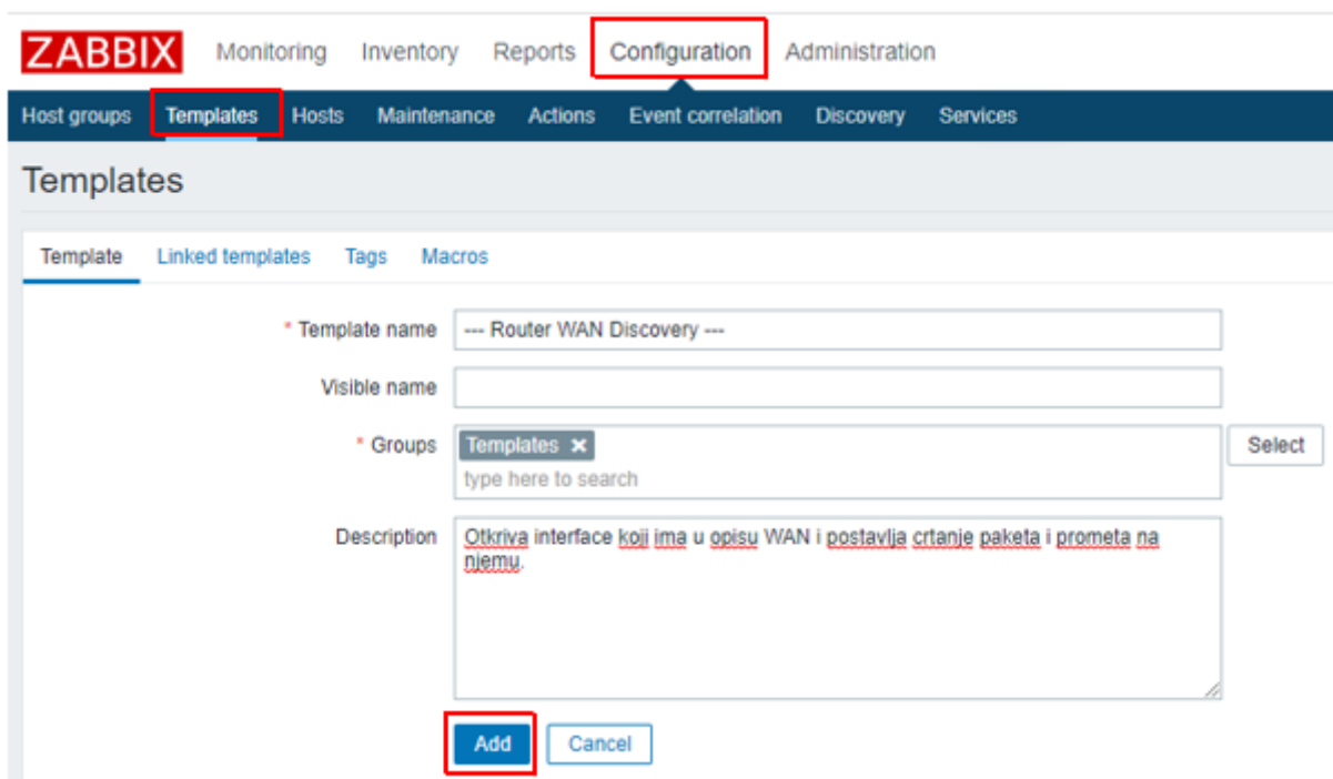
Slika 29 Prikaz postavljanja naziva i opisa predloška
