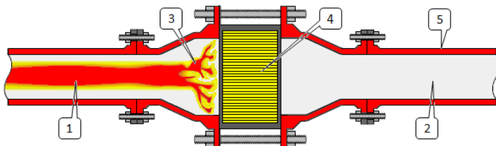
Slika 27. Prikaz hvatača plamena (1 – strana izložena plamenu; 2- šticeana strana; 3 – plamen stabiliziran na hvataču plamena; 4- hvatač plamena apsorbira toplinu i gasi plamen; 5 – cijev) Izvor: [42]
