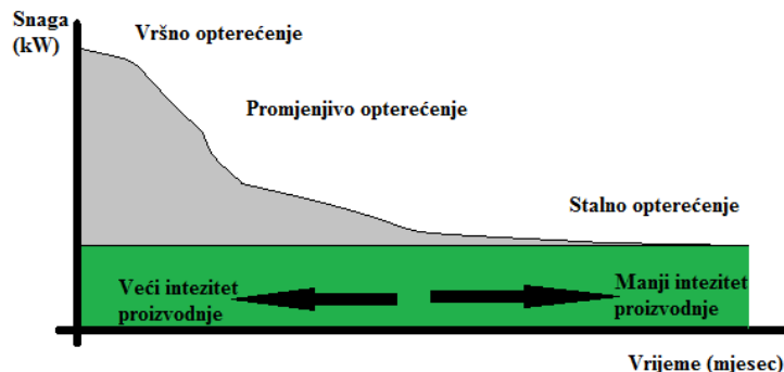
Dijagram 5. Krivulja trajanja opterećenja
