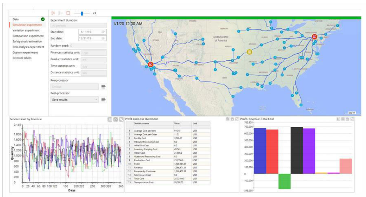
Slika 10 Softver anyLogistix
