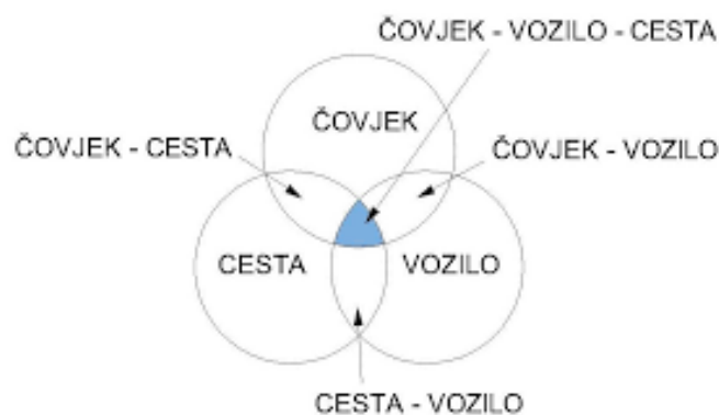
Slika 1. Venov dijagram
