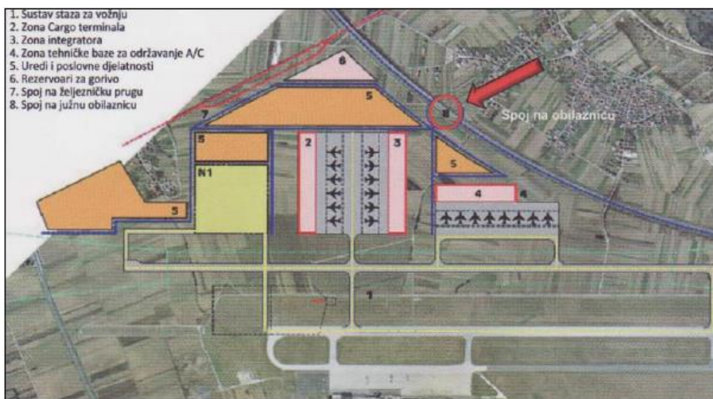
Slika 16. Master plan zračne luke Zagreb, [23]
