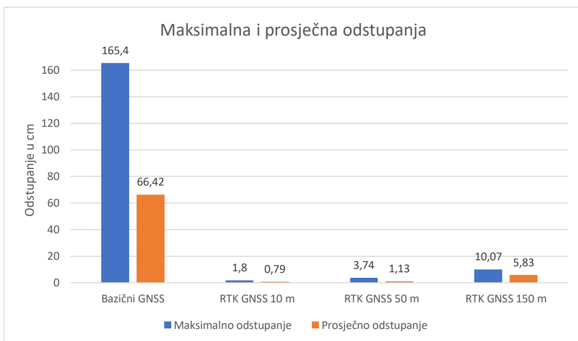
Grafikon 2. Usporedba maksimalnih i prosječnih odstupanja od referentne lokacije bazičnog GNSS-a i RTK GNSS-a (stanice udaljene 10, 50 i 150 m)
