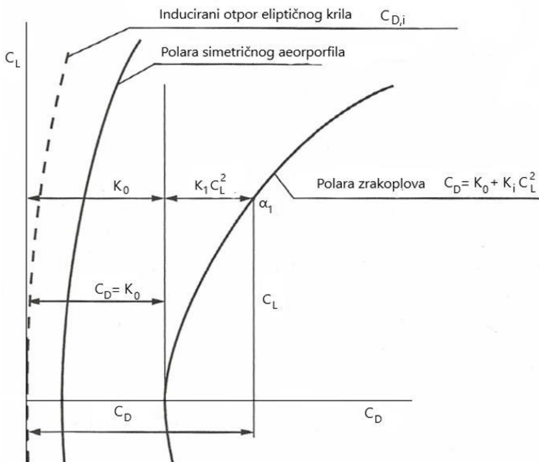
Slika 1. Grafički prikaz polare zrakoplova [1]
