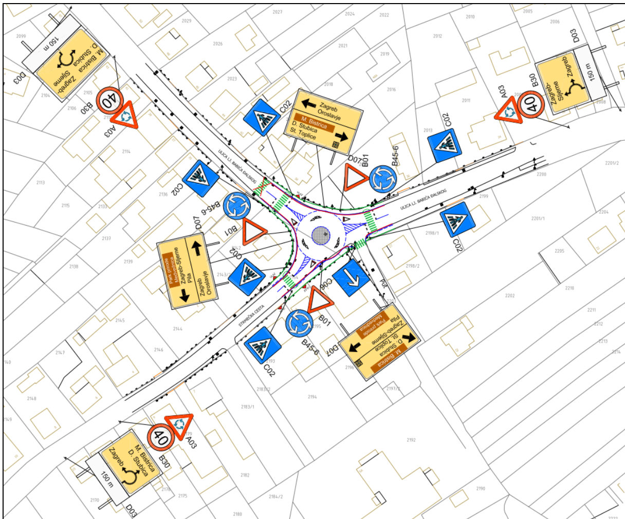
Slika 24: Situacija signalizacije predmetnog raskrižja [21]
