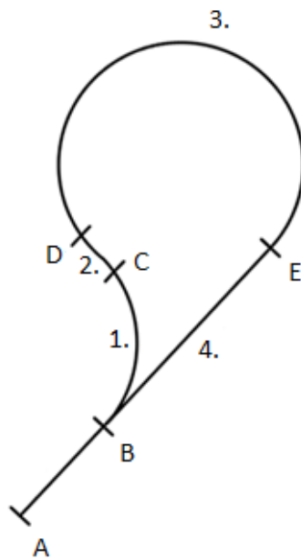
Slika 15. Proceduralni zaokret 80^\circ/260^\circ i njegovi segmenti
