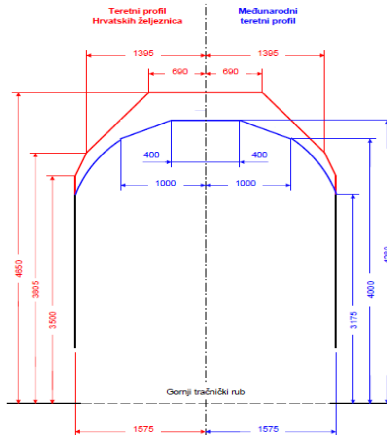
Slika 20. Teretni profil
